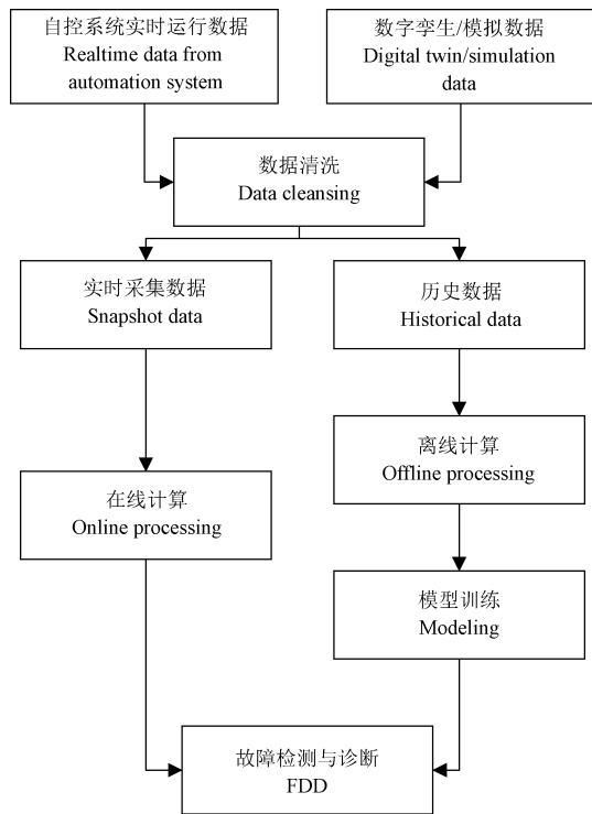
图 2 常见的机器学习 FDD 方法流程
